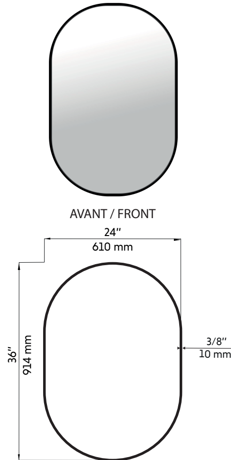
ARRIÈRE / BACK
