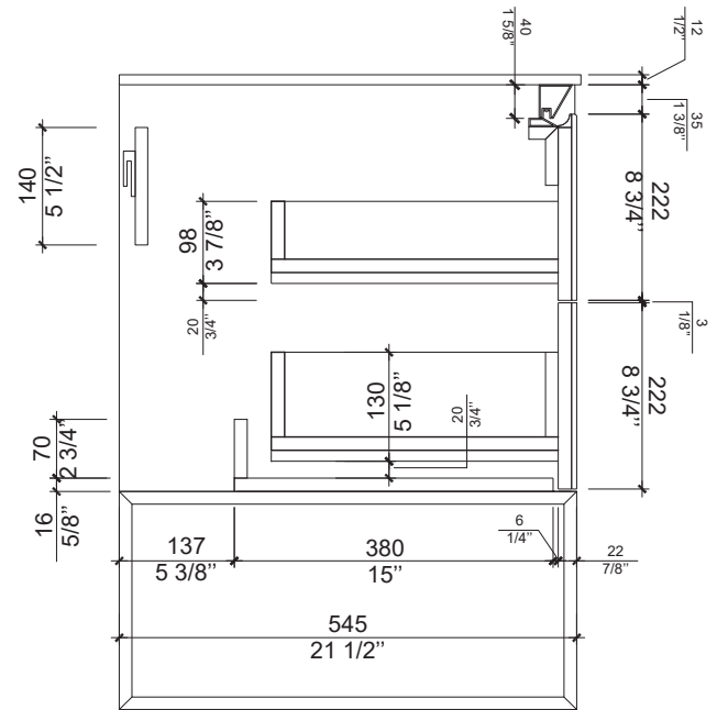
Élévation latérale / Side elevation
