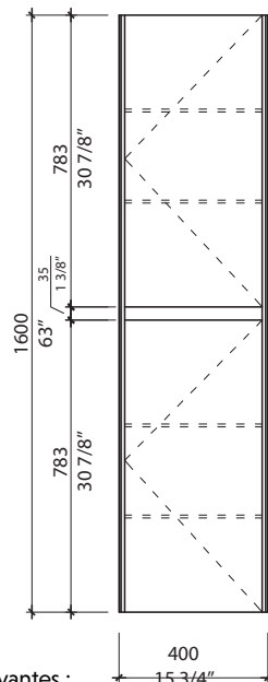
Vu de devant Front view
