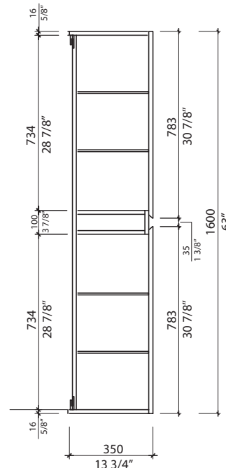
Élévation latérale Side elevation
