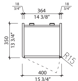
Vu de dessus Top view
