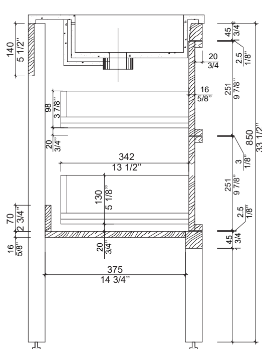
Élévation latérale Side elevation
