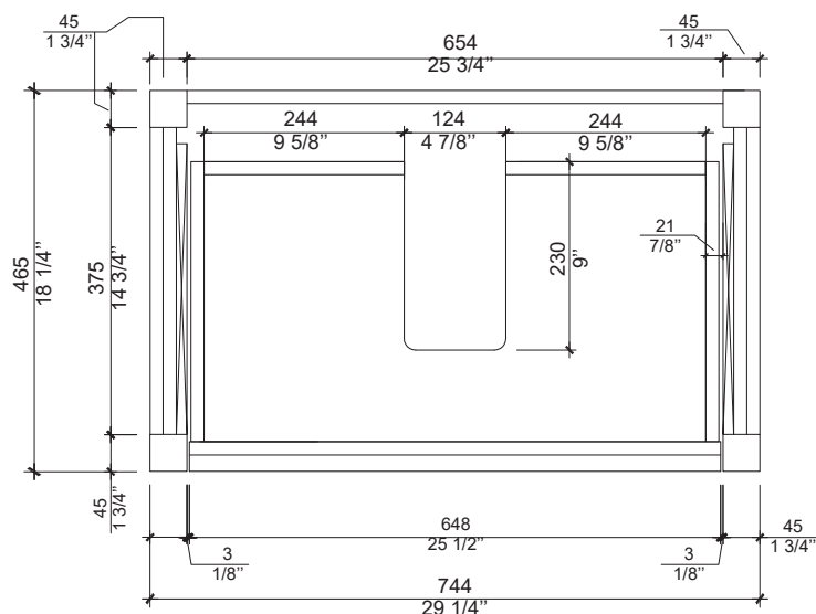
Détail du plan du tiroir du haut Top drawer plan detail
