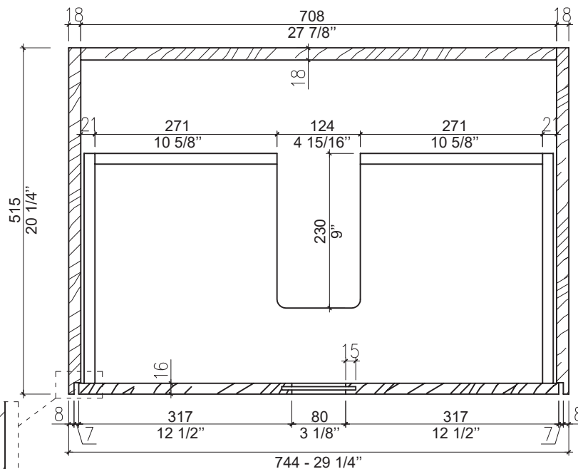
Détail du plan du tiroir du haut Top drawer plan detail
