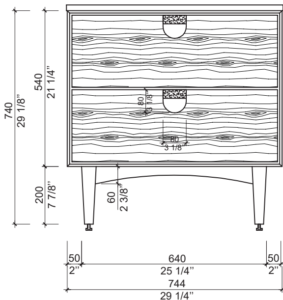
Vu de devant / Front view
