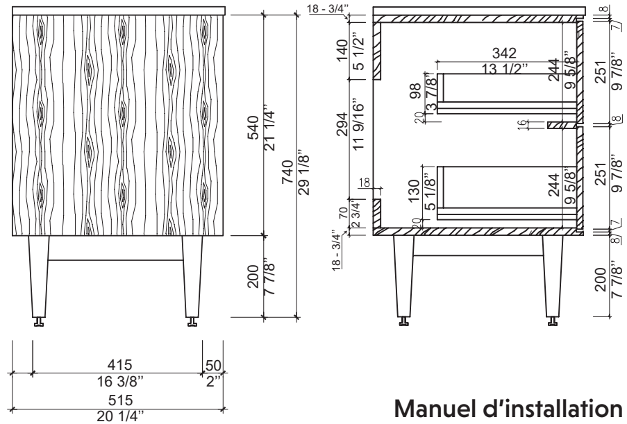
Élévation latérale / Side elevation
