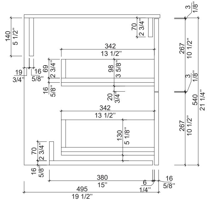
Élévation latérale / Side elevation
