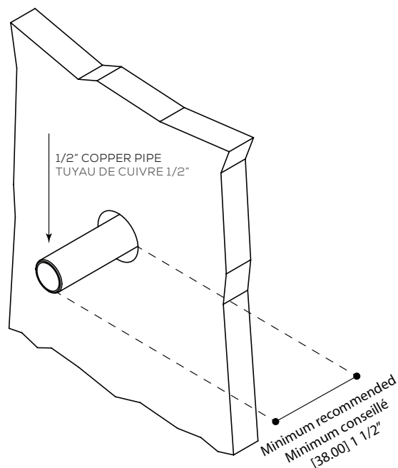
SLIP-FIT TUB SPOUT RECOMMENDATIONS RECOMMANDATIONS POUR LE BEC DE BAIN « SLIP-FIT »
